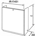
配管カバーH32K450
